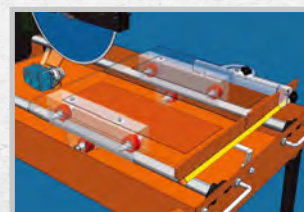
Подвижный рабочий стол оснащен восьмью (8-ю) шарикоподшипниками
